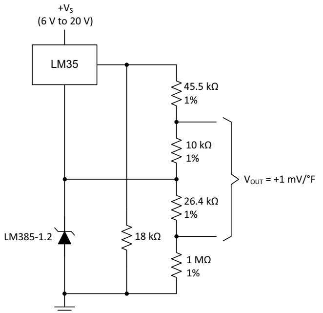
Figure 21. Fahrenheit Thermometer
