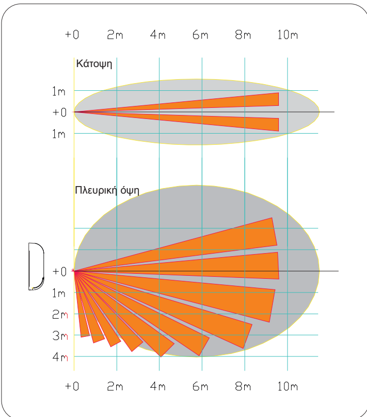
ΔΙΑΓΡΑΜΜΑ ΚΑΛΥΨΗΣ ΑΝΙΧΝΕΥΤΗ
