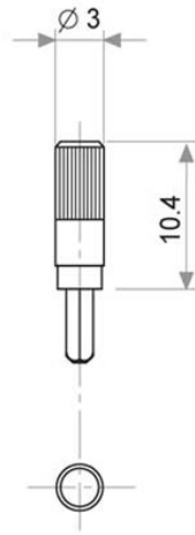
5016 PT10 Trimmer
